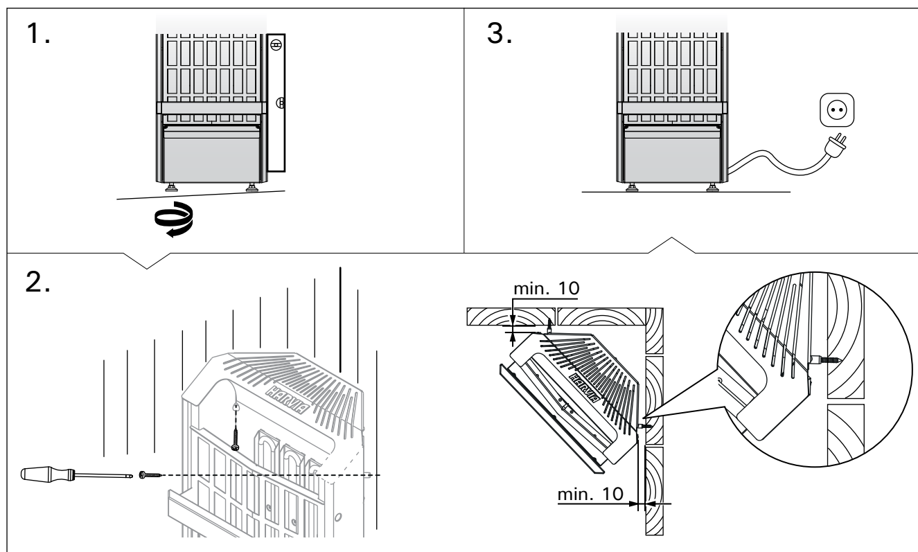
Рисунок 4. Установка каменки
