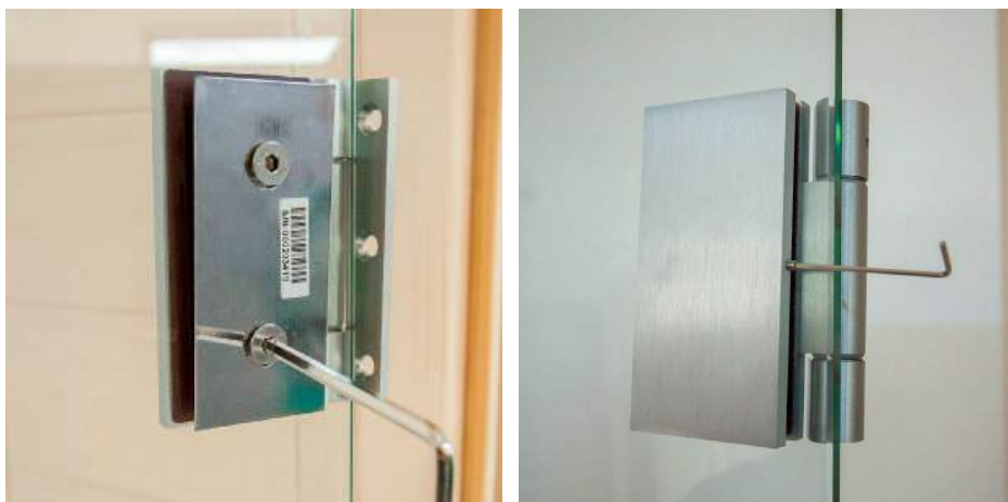
Fig. 32: Montagem das ferragens da porta 2
