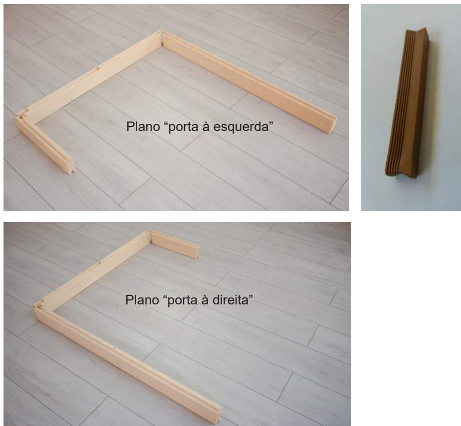
Fig. 1: Instalação dos três elementos da armação do chão
