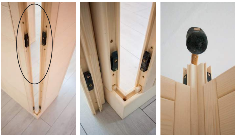
Fig. 4 : Raccorder les éléments muraux avec les montants d'angle
