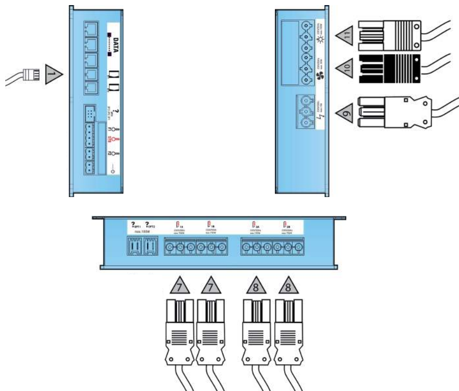
Abb. 26: Anschlüsse Leistungsteil
