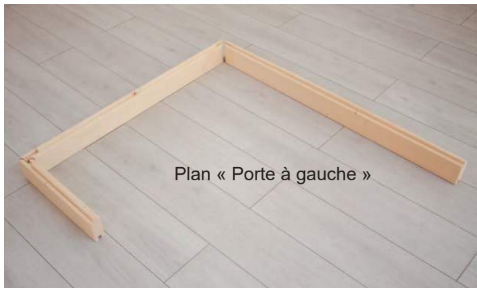
Fig. 1 : Pose des trois éléments de cadre de plancher
